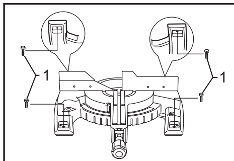
► 1. Bolts
