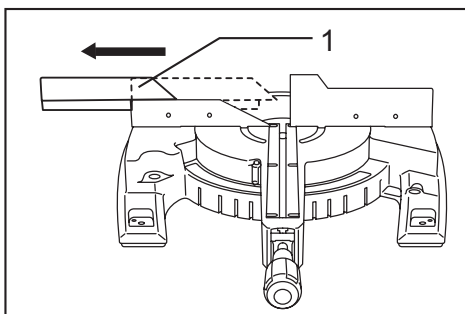
► 1. Sliding fence
